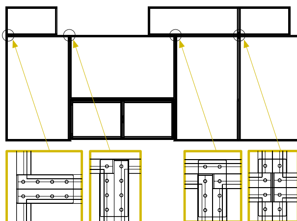
Fissaggio con piastre
